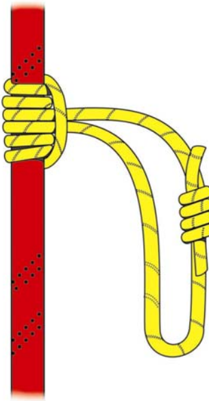
Figure 6-9. Prusik Hitch
